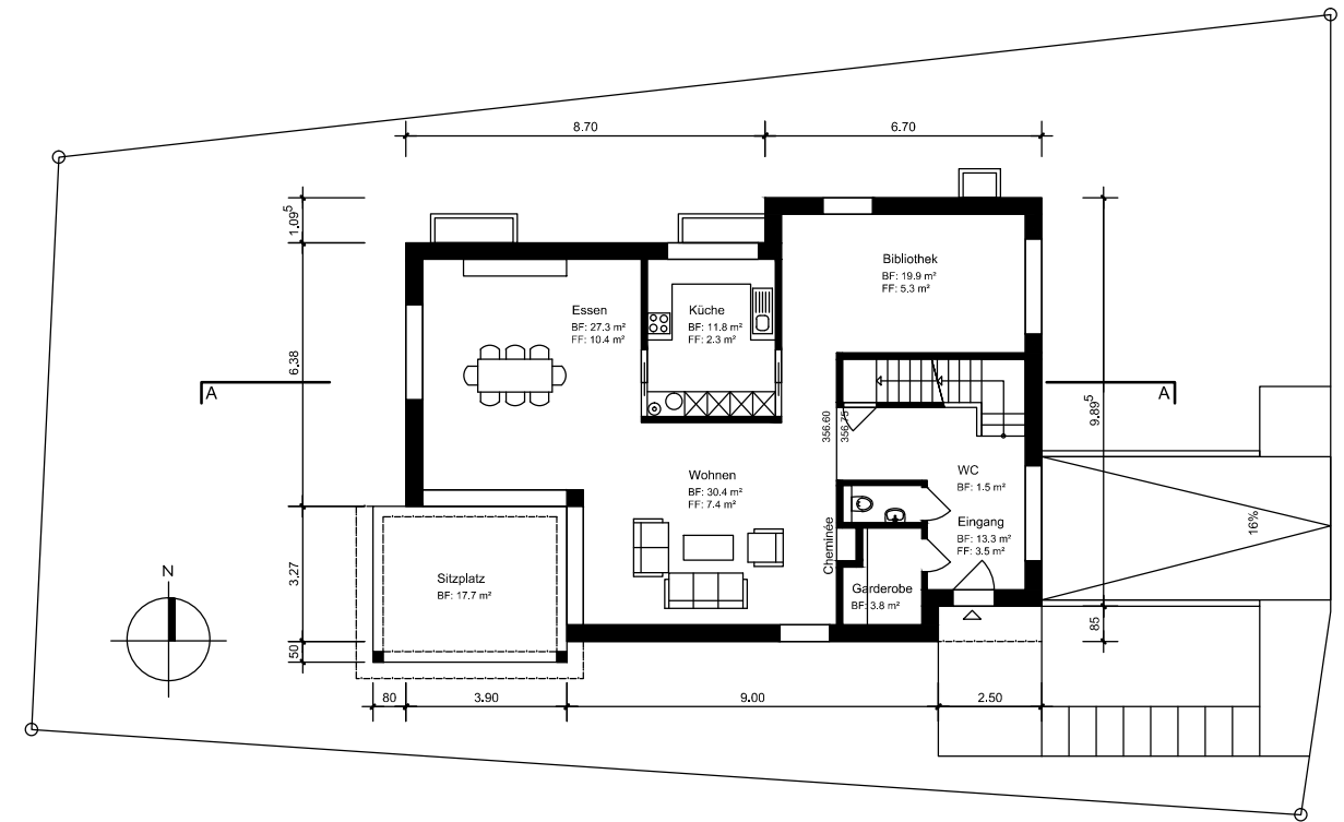
ERDGESCHOSS
