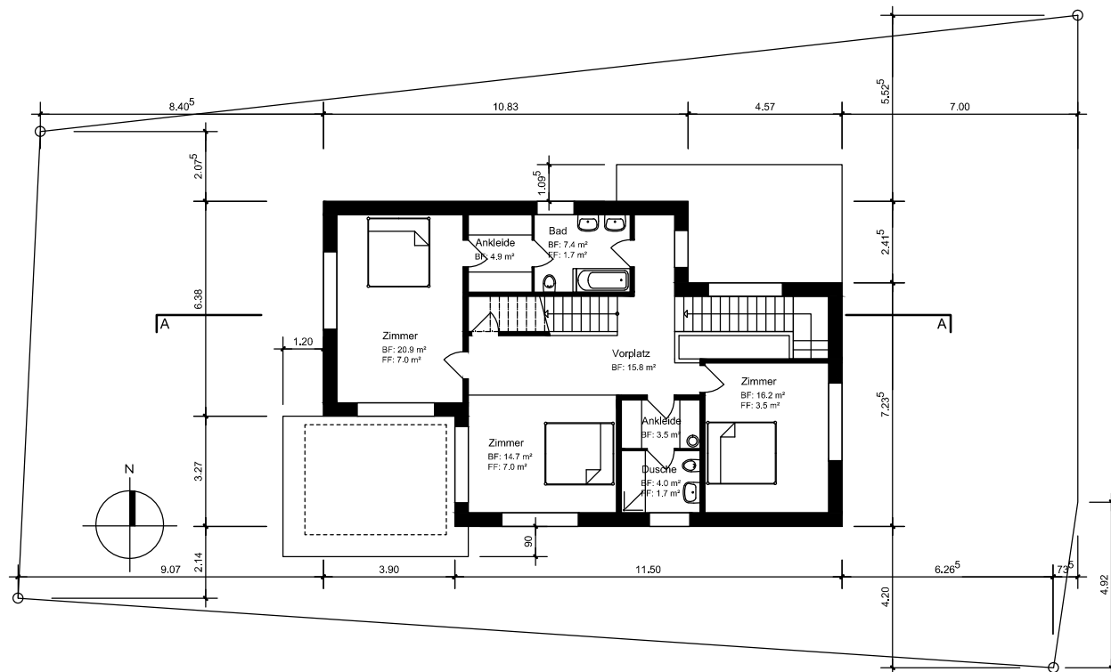
OBERGECHOSS
