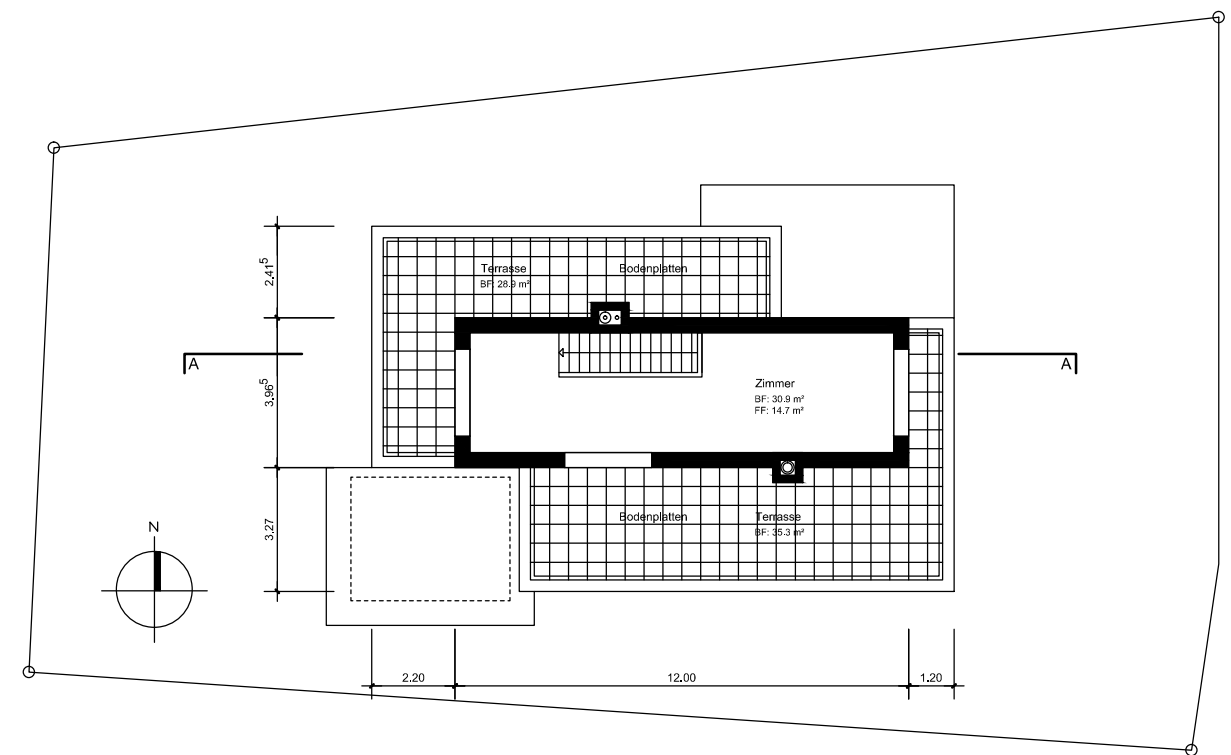
DACHGESCHOSS
