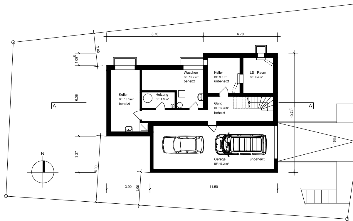
UNTERGESCHOSS
